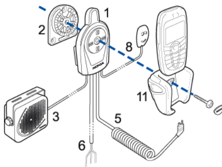
Instalacija za automobil s pasivnim držačem mobilnog telefona
