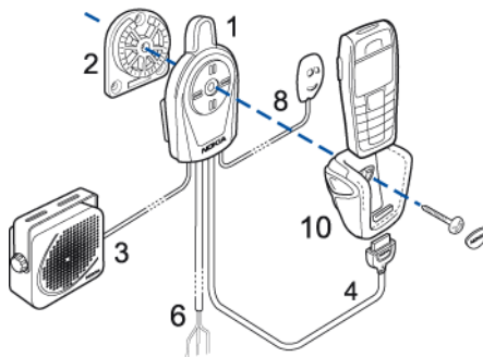
Instalacija za automobil s aktivnim držačem mobilnog telefona
